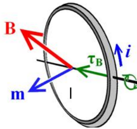
Fig. 3 - Espira com corrente elétrica imersa em um campo magnético sofre torque magnético.
