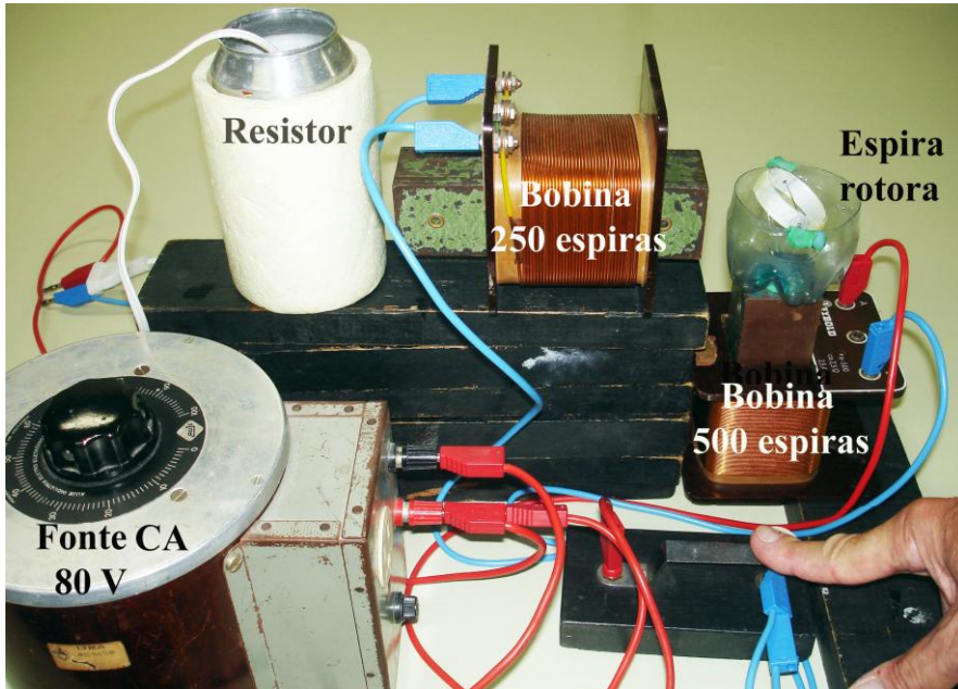
Fig. 6 - Motor de indução monofásico com resistor em série com uma das bobinas.
