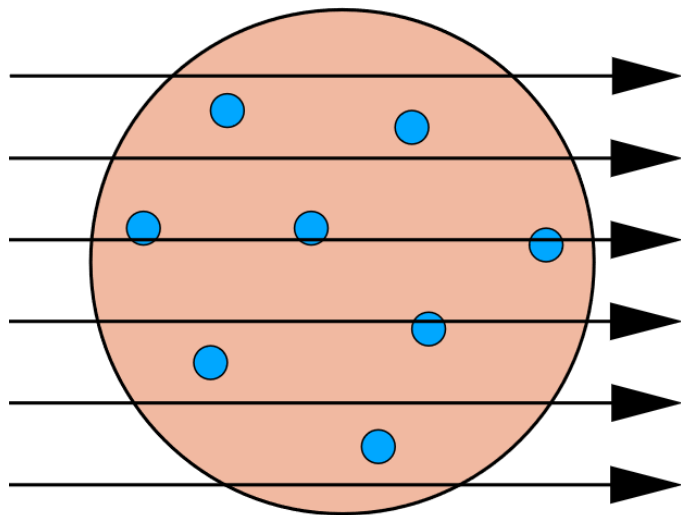
MODELO THOMSON
