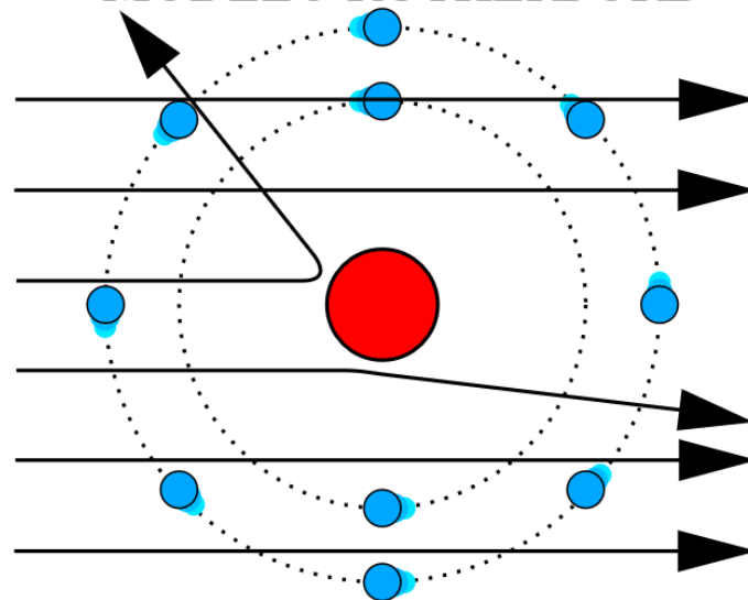
MODELO RUTHERFORD
